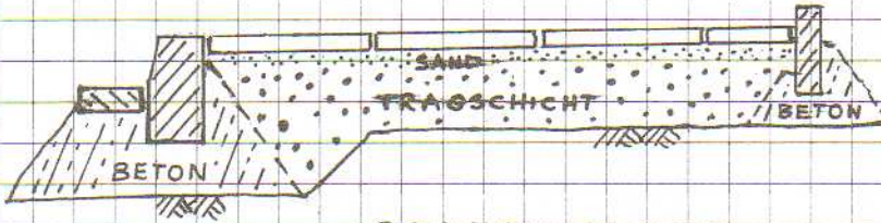
SCHNITT M 1:20
